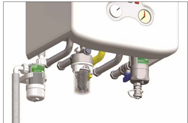
Esempio di installazione di: Neutralizzatore, filtro dosatore PolyFAR e defangatore CompactFAR sotto una caldaia domestica.
