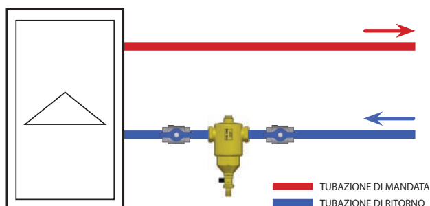
CORRETTA INSTALLAZIONE DEL DEFANGATORE NEGLI IMPIANTI GENERICI
